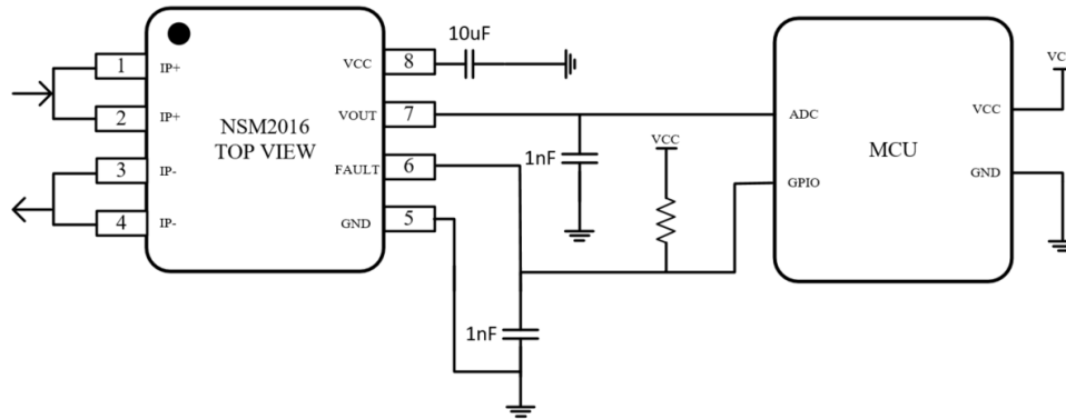
Figure 6.1 NSM2016 典型应用电路
