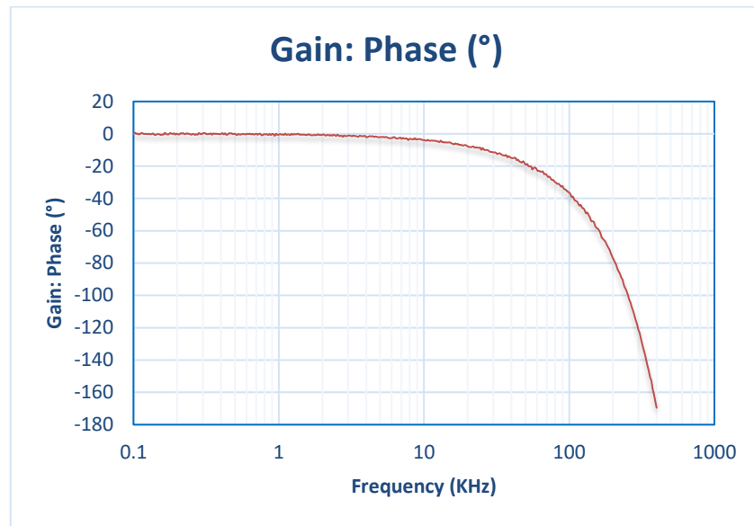
Figure 5.4 NSM2016 相频响应曲线
