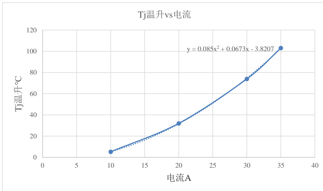
Figure 6.4 NSM2016 在不同电流下结温曲线预估函数(PCB 在 worst case)
