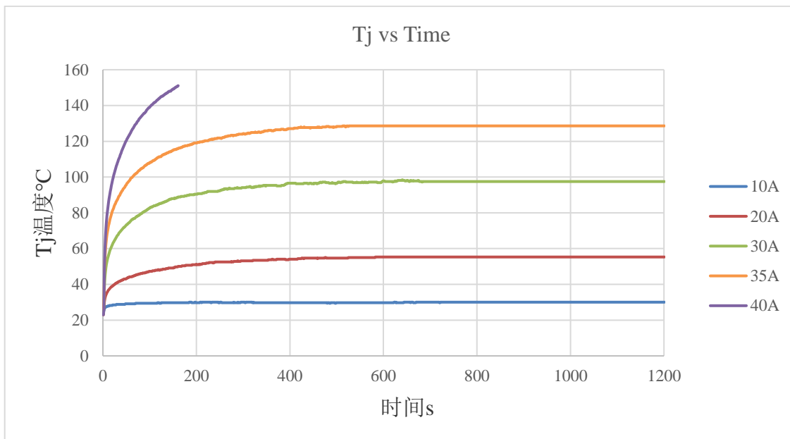
Figure 6.3 NSM2016 在不同电流下结温曲线
