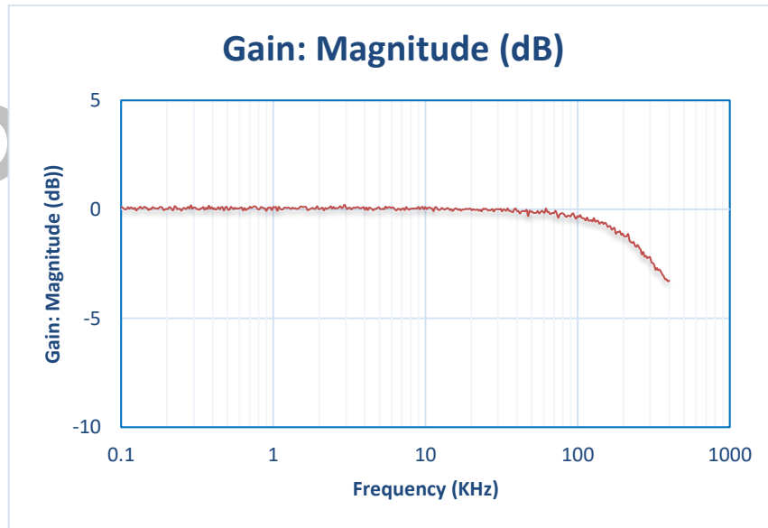
Figure 5.3 NSM2016 幅频响应曲线
