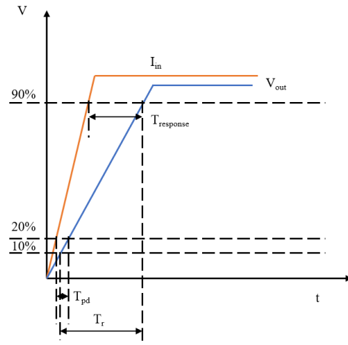
Figure 5.6 NSM2016 响应时间定义
