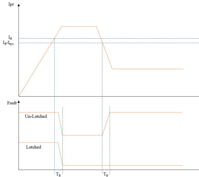
Figure 5.2 NSM2016 过流 Latch 表现
